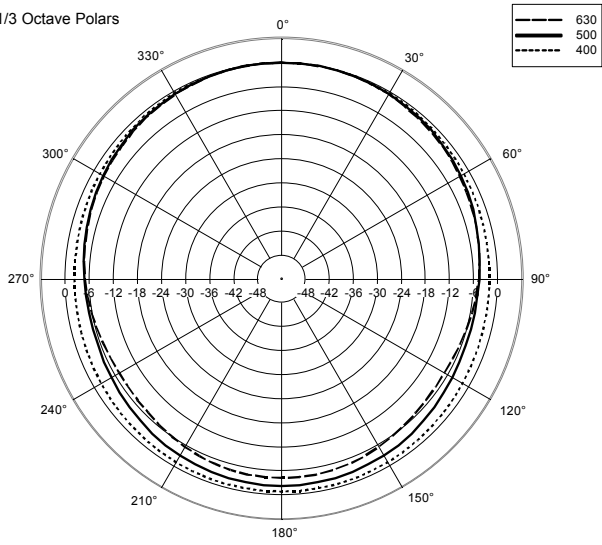
1/3 Octave Polars
